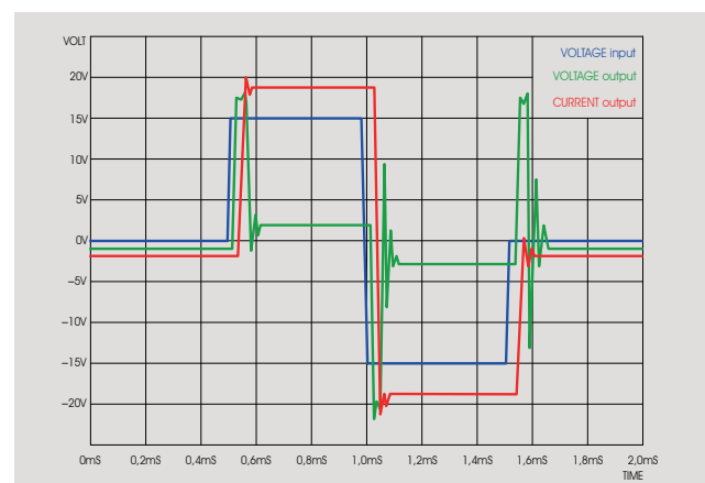
Abb. 2: iTRON AA Stromverstärker Simulation an 2 Wege Box
